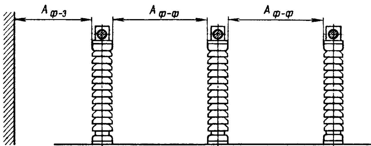
Рис. 4.2.1. Наименьшие расстояния в свету при жестких шинах между токоведущими и заземленными частями ( A_{\phi-з} ) и между токоведущими частями разных фаз ( A_{\phi-φ} )
