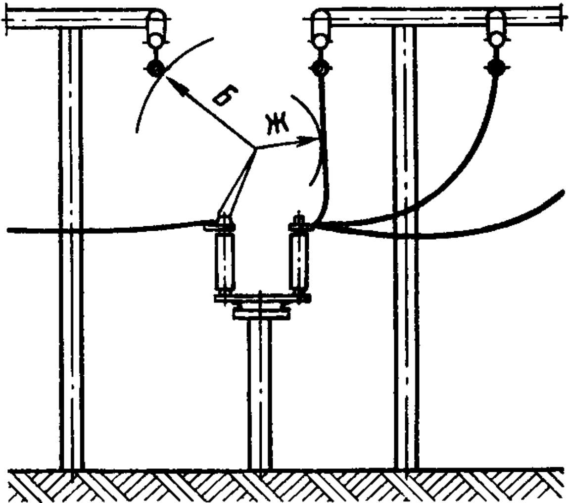
Рис. 4.2.9. Наименьшие расстояния от контактов и ножей разъединителей в отключенном положении до заземленных и токоведущих частей
