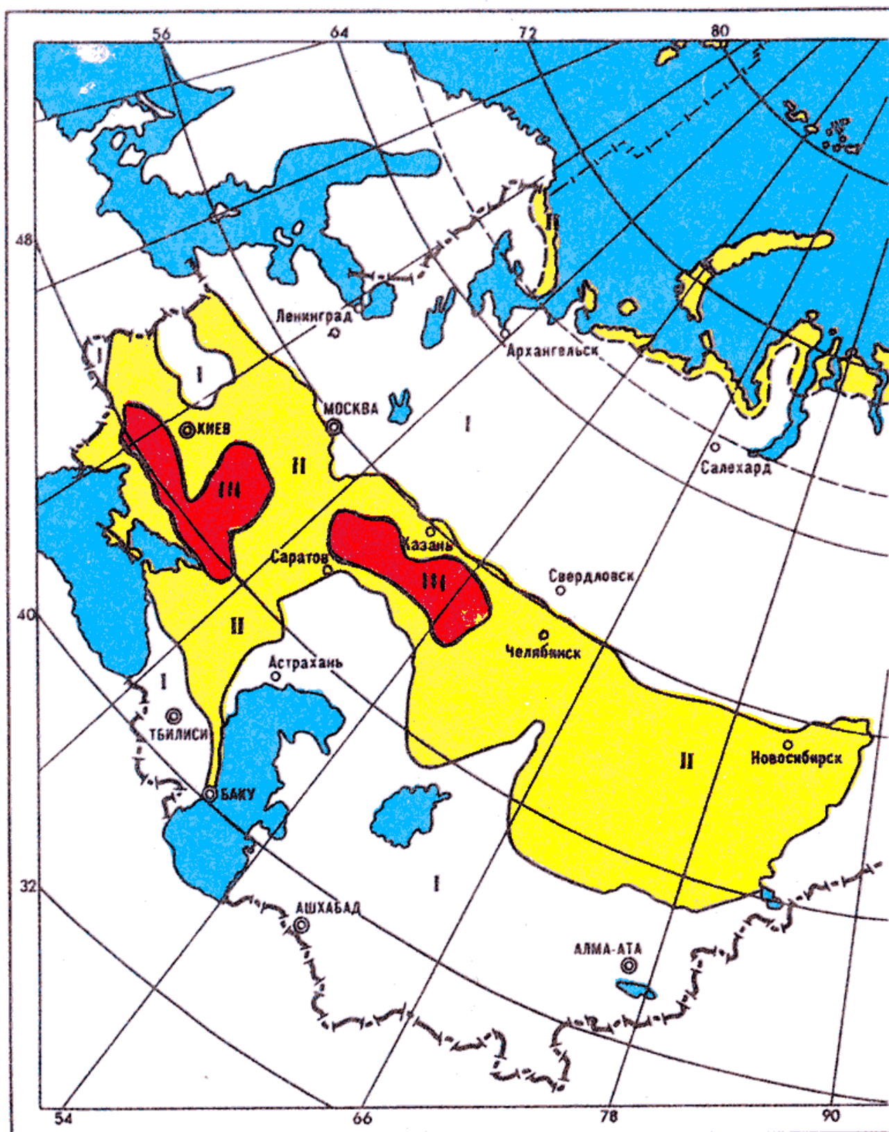
Рис. 2.5.11. Карта районирования территории по пляске проводов. Лист 1
