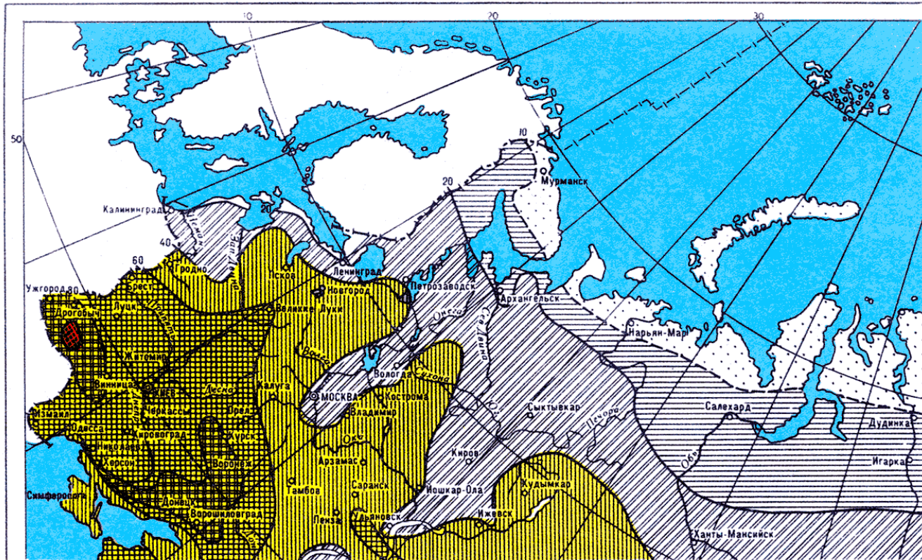
Рис. 2.5.13. Карта среднегодовой продолжительности гроз. Лист 1
