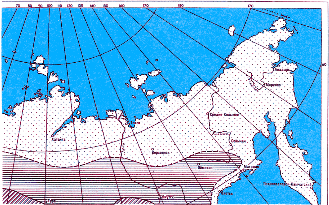
Рис. 2.5.15. Карта среднегодовой продолжительности гроз. Лист 3
