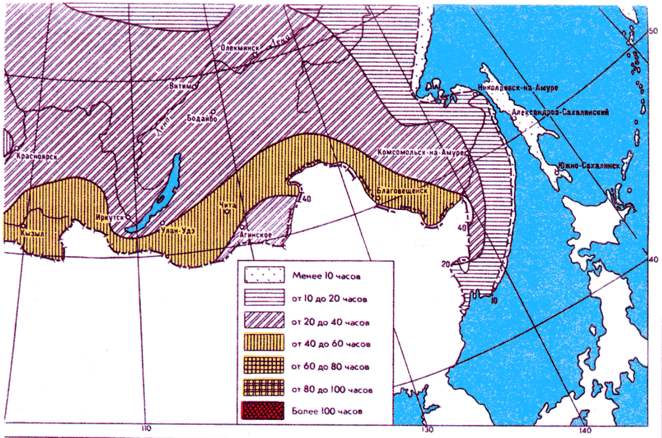
Рис. 2.5.16. Карта среднегодовой продолжительности гроз. Лист 4
