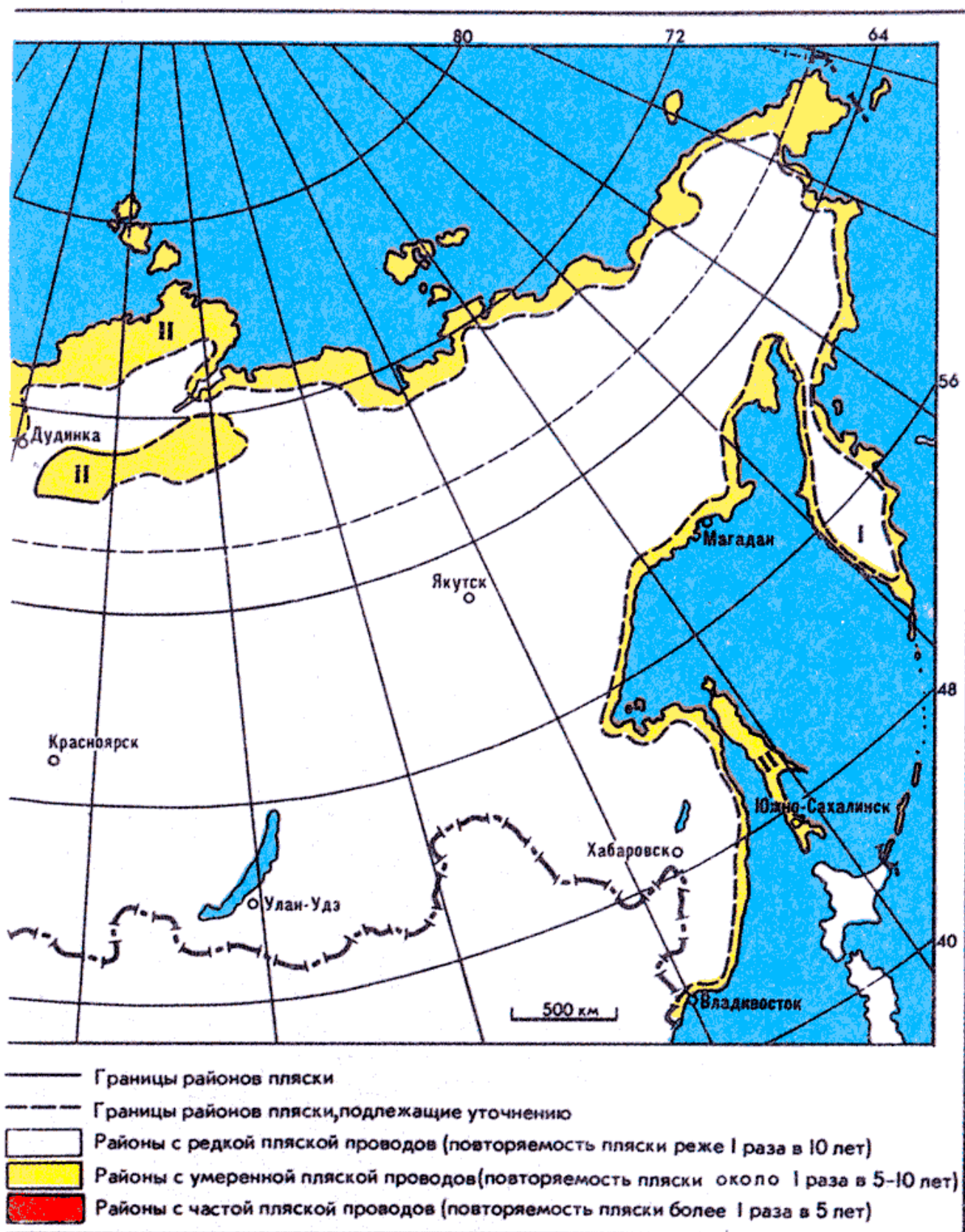
Рис. 2.5.12. Карта районирования территории по пяске проводов. Лист 2
