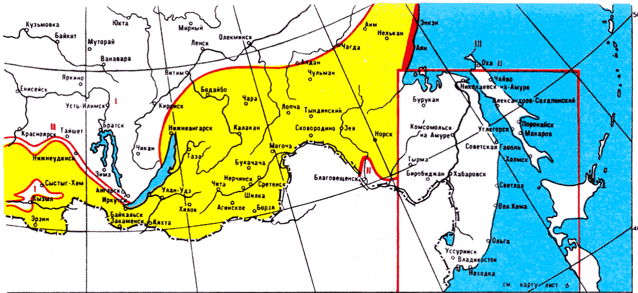
Рис. 2.5.7. Карта районирования территории по толщине стенки гололеда. Лист 3
