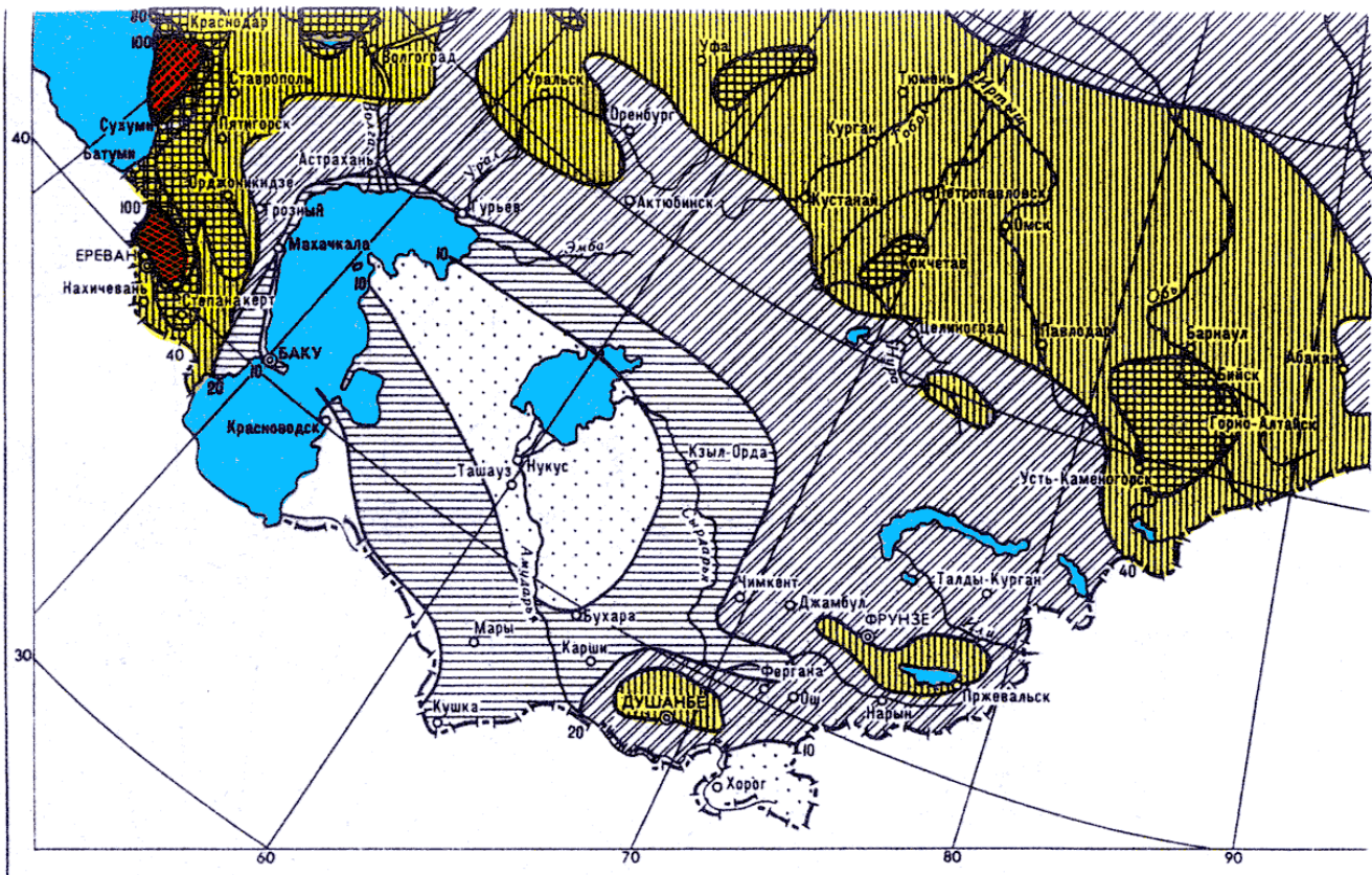
Рис. 2.5.14. Карта среднегодовой продолжительности гроз. Лист 2
